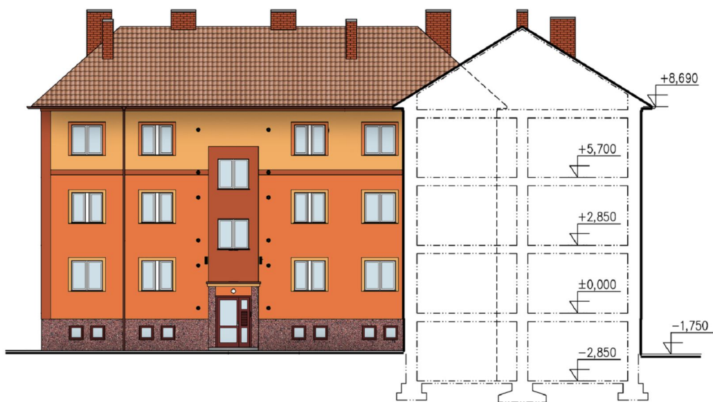
POHLED DVORNÍ (SV)
